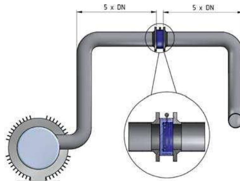
(Abb.1 / pic.1) Leitungsbeispiel / Pipeline example
